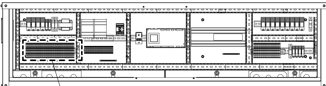
Position boîte à bornes auxiliaire
