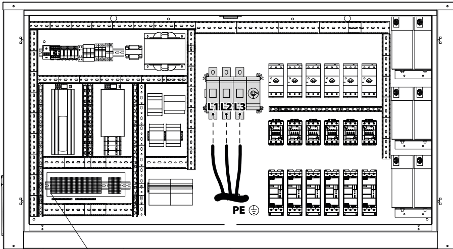
Boîte à bornes auxiliaire
