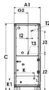
MODULE ELITE®
