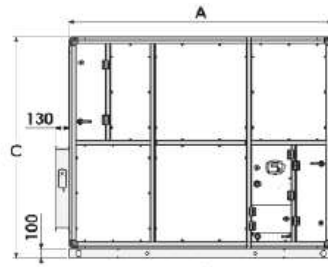
EXAECO® 10 et 13
