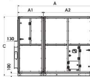
EXAECO® 17 et 22
